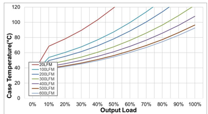
图 4: 工作亮温 VS 输出负载(满载)
