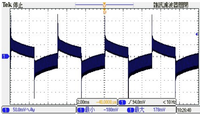
图 7: 进阶负载的输出变化
