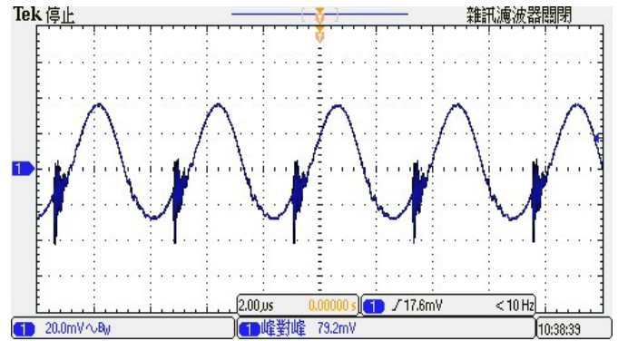
图 8: 输出电压纹波与噪声(满载).
