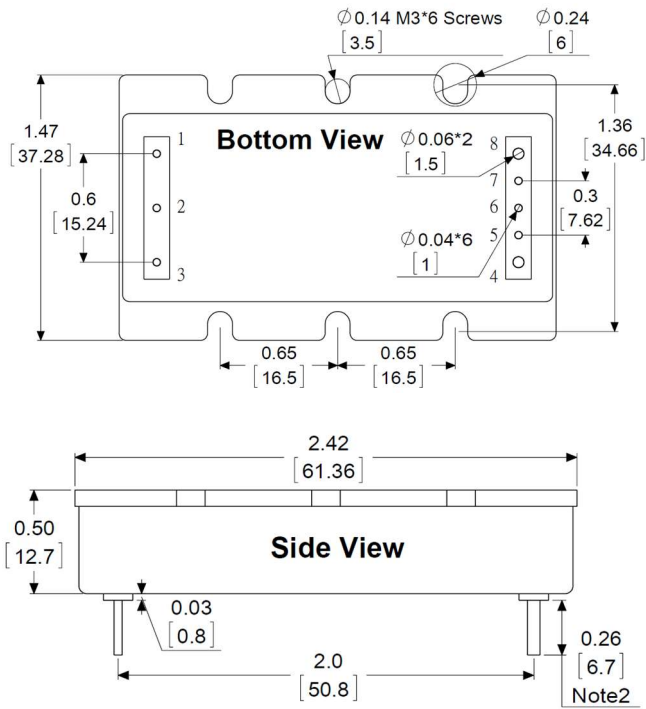
尺寸图 - B (金属壳法兰片 Vicor 引脚)
